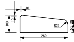
低下縁石
