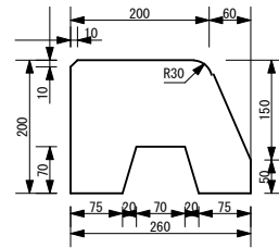
標準縁石
