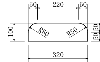
低下縁石
