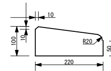
低下縁石
